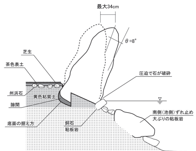
模式図 (西側立面図)
