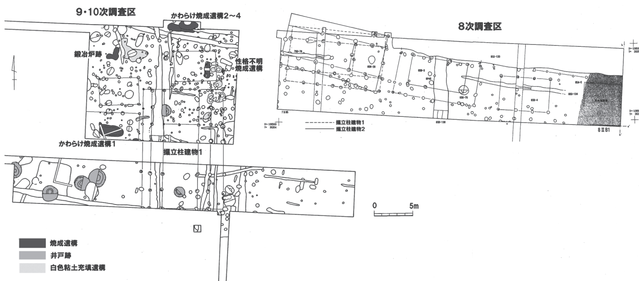
図2 白鳥館遺跡第10次調査区平面図
