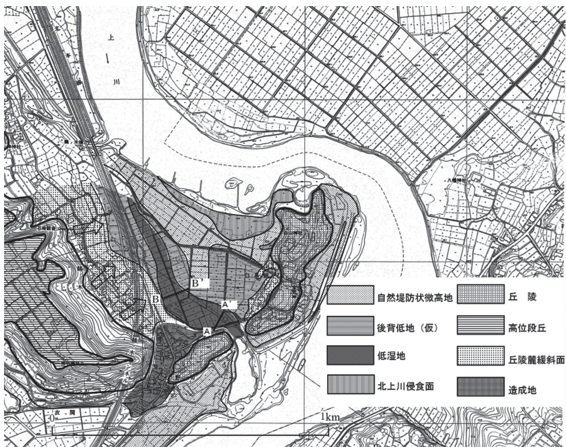
図3 白鳥館西方の地形面分類図
