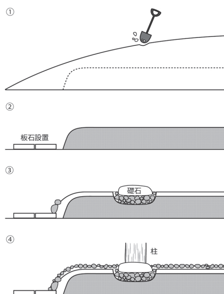
本堂基壇の作り方模式図（案）
