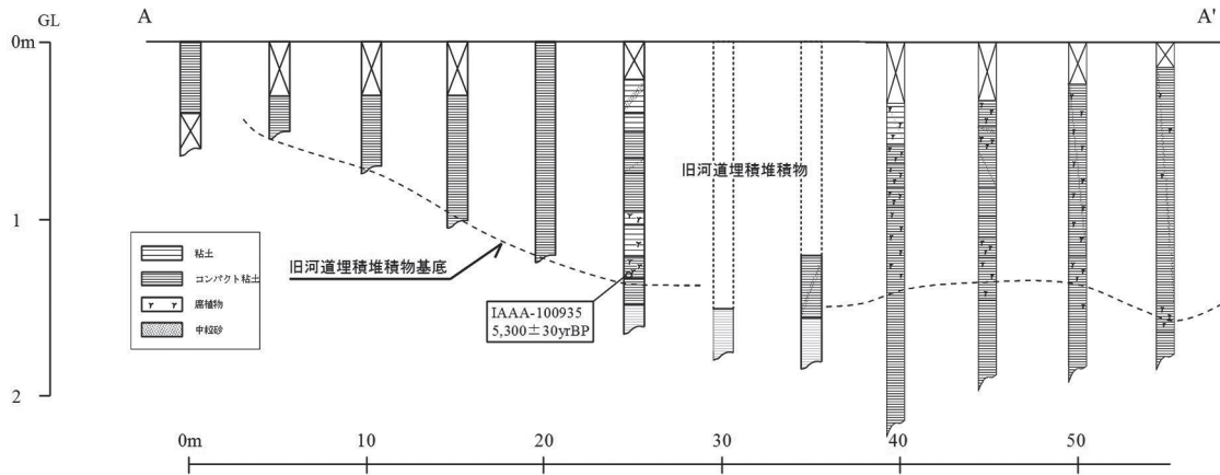
図4 白鳥館西方の地形面における河川跡調査断面図 (A - A')
