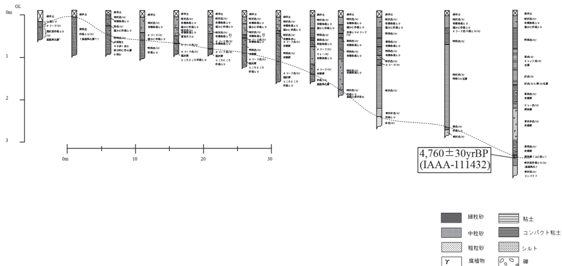
図5 白鳥館西方の地形面における河川跡調査断面図 (B - B')
