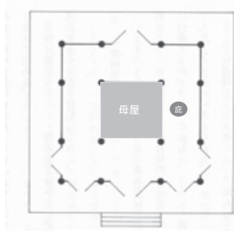
一間四面堂の平面 図7
